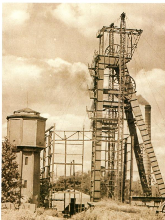
Důl Kohinoor II., Mariánské Radčice, stavba skipové těžní věže, Koh 04
